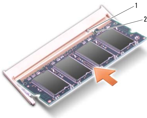
1 выступ 2 паз
